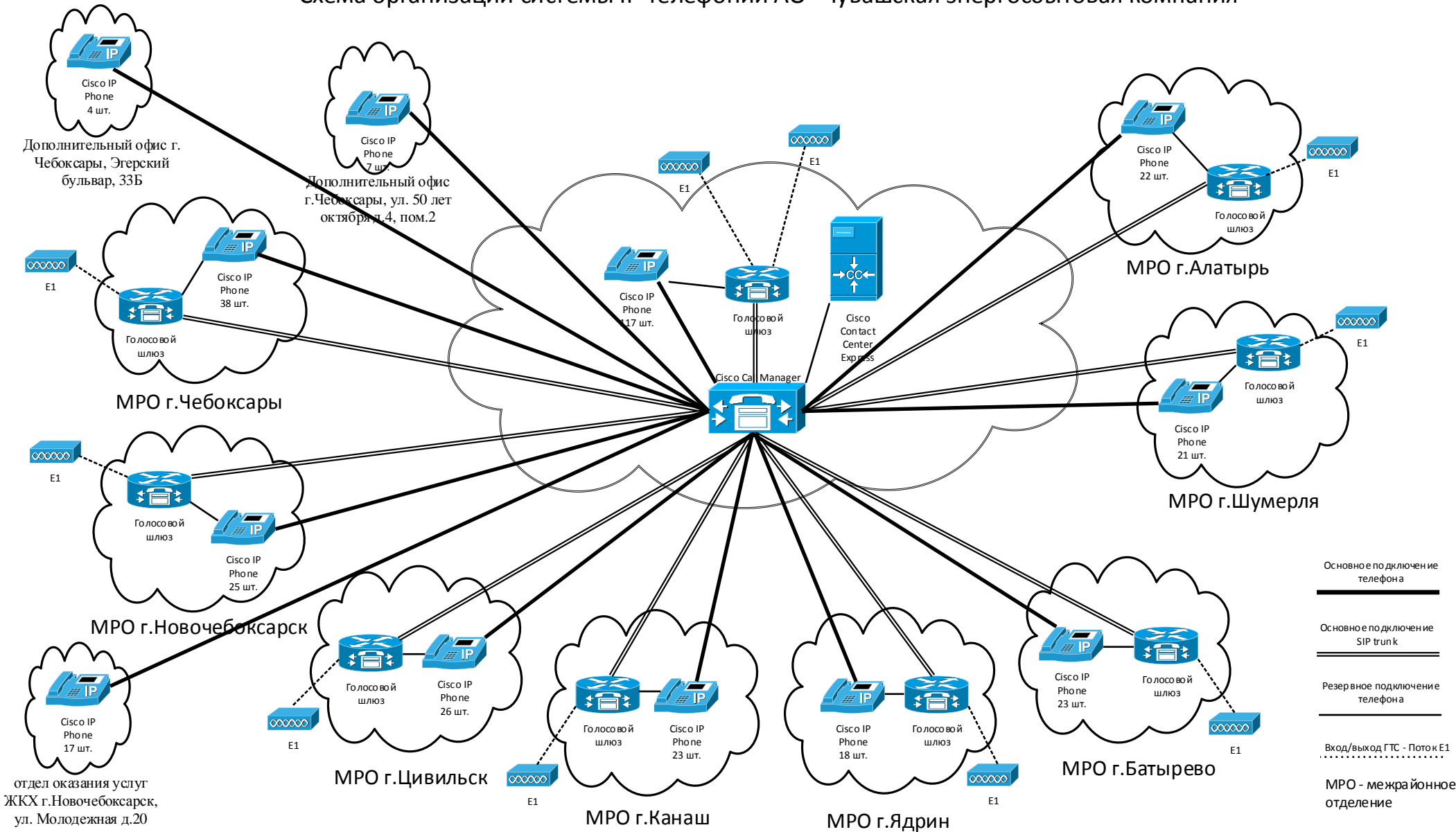
Схема организации системы IP-телефонии АО “Чувашская энергосбытовая компания”
